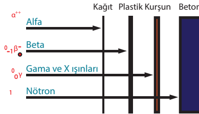
Şekil 1: Radyasyon Tiplerine Göre Uygulanan Zırhlamalar
